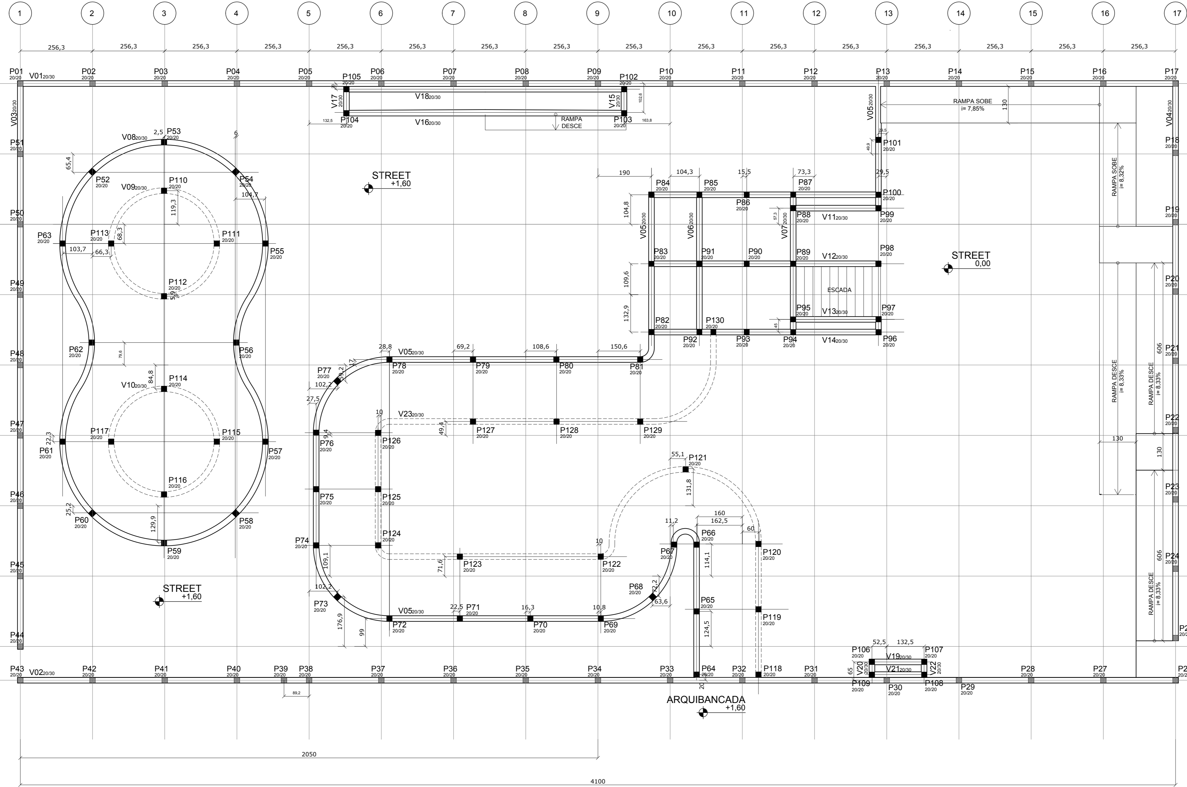
PLANTA DE FÔRMAS E LOCAÇÃO TOPO DA PISTA ESCALA.....1/75
