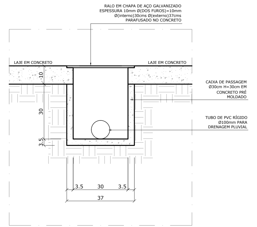
DETALHE 03 CAIXA DE PASSAGEM E TUBO DE PVC RÍGIDO EM CORTE ESCALA..... 1/10
