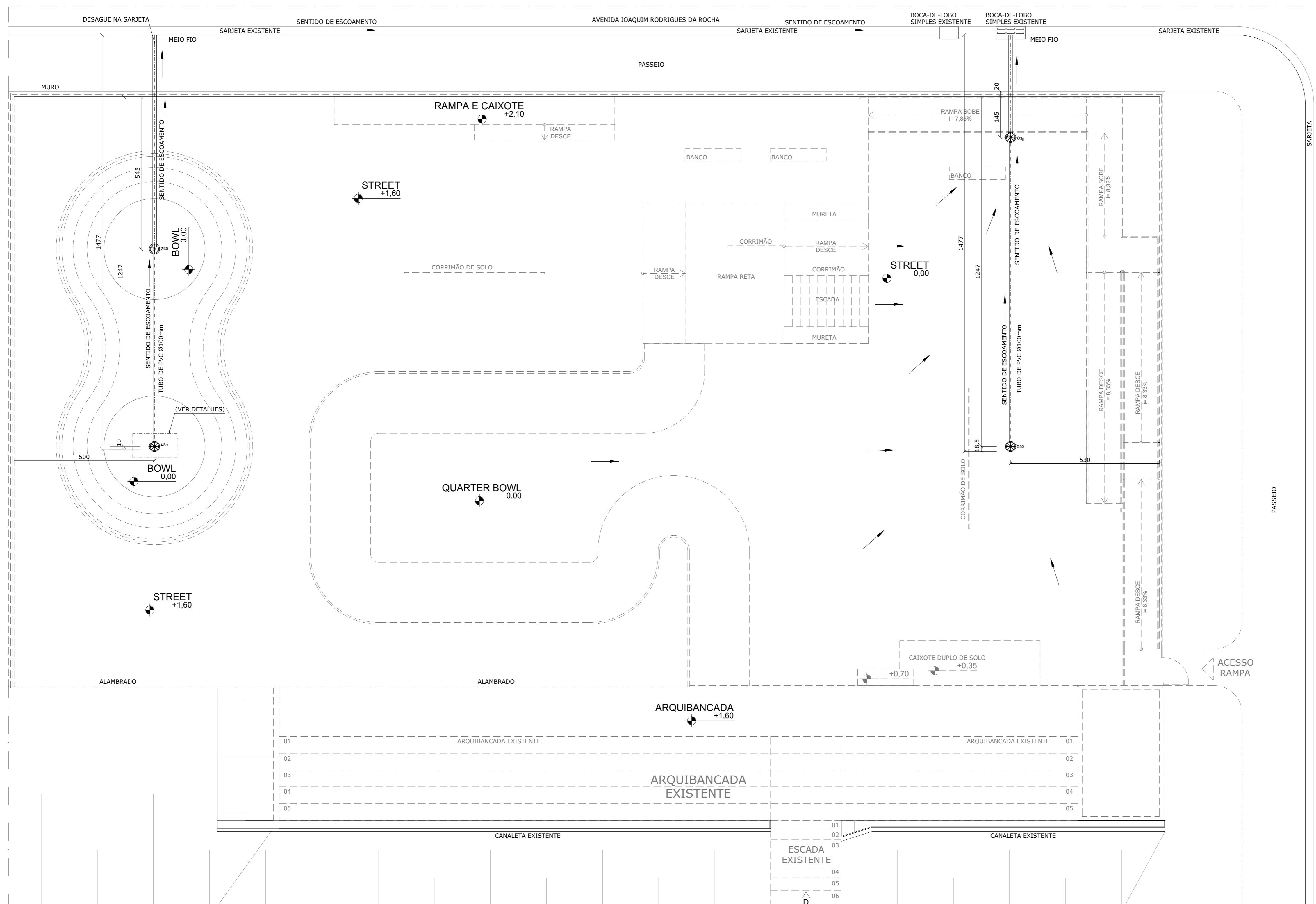
IMPLANTAÇÃO DE DRENAGEM ESCALA..... 1/75
