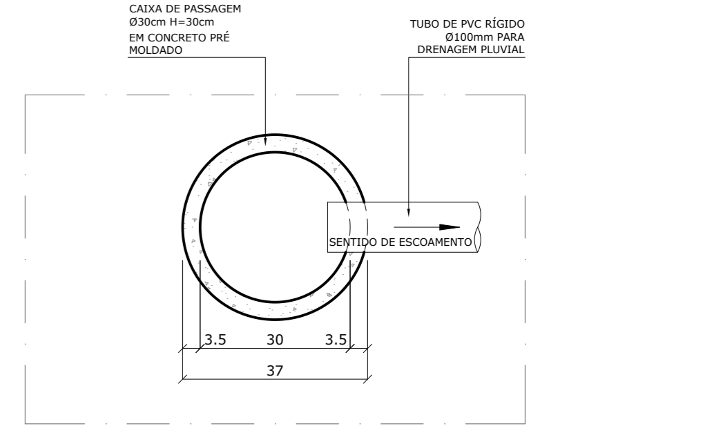
DETALHE 02 CAIXA DE PASSAGEM E TUBO DE PVC RÍGIDO EM PLANTA ESCALA..... 1/10
