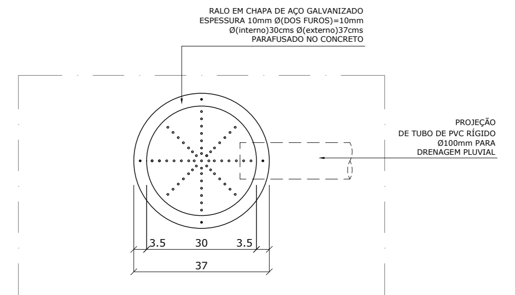
DETALHE 01 VISTA SUPERIOR - RALO ESCALA..... 1/10
