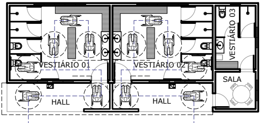
PLANTA DE CIRCULAÇÃO - ACESSIBILIDADE ESCALA..... 1/50
