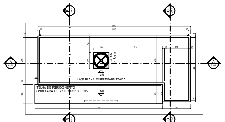
PLANTA DE COBERTURA ESCALA..... 1/100
