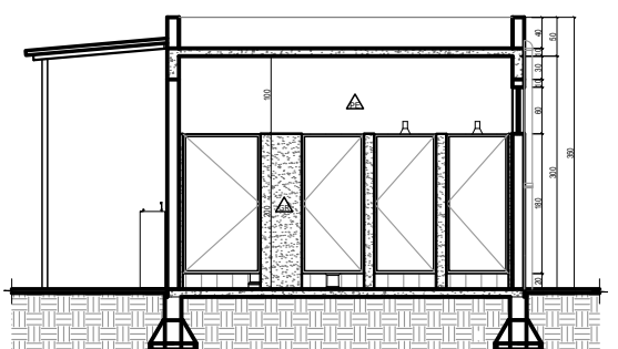
CORTE BB ESCALA..... 1/50
