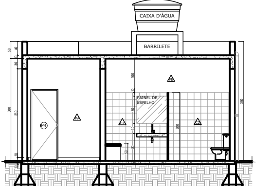
CORTE CC ESCALA..... 1/50
