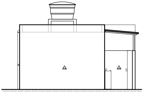
FACHADA LATERAL DIREITA ESCALA..... 1/50
