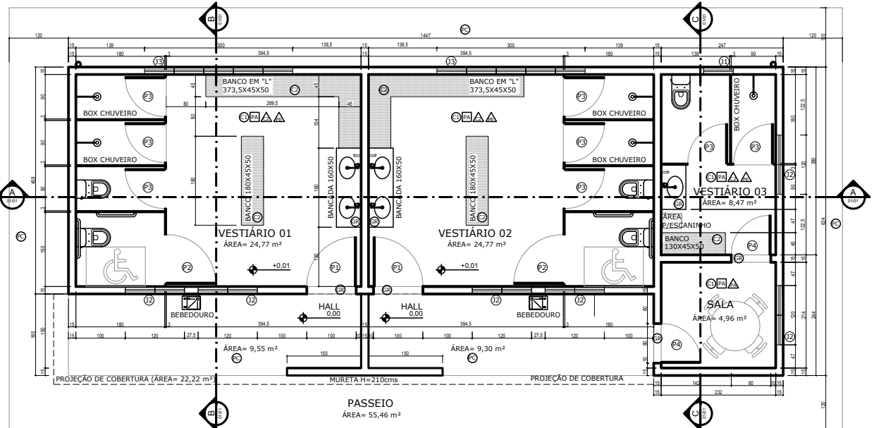
PLANTA VESTIÁRIO ÁREA TOTAL=92,97 m 2 ESCALA..... 1/50
