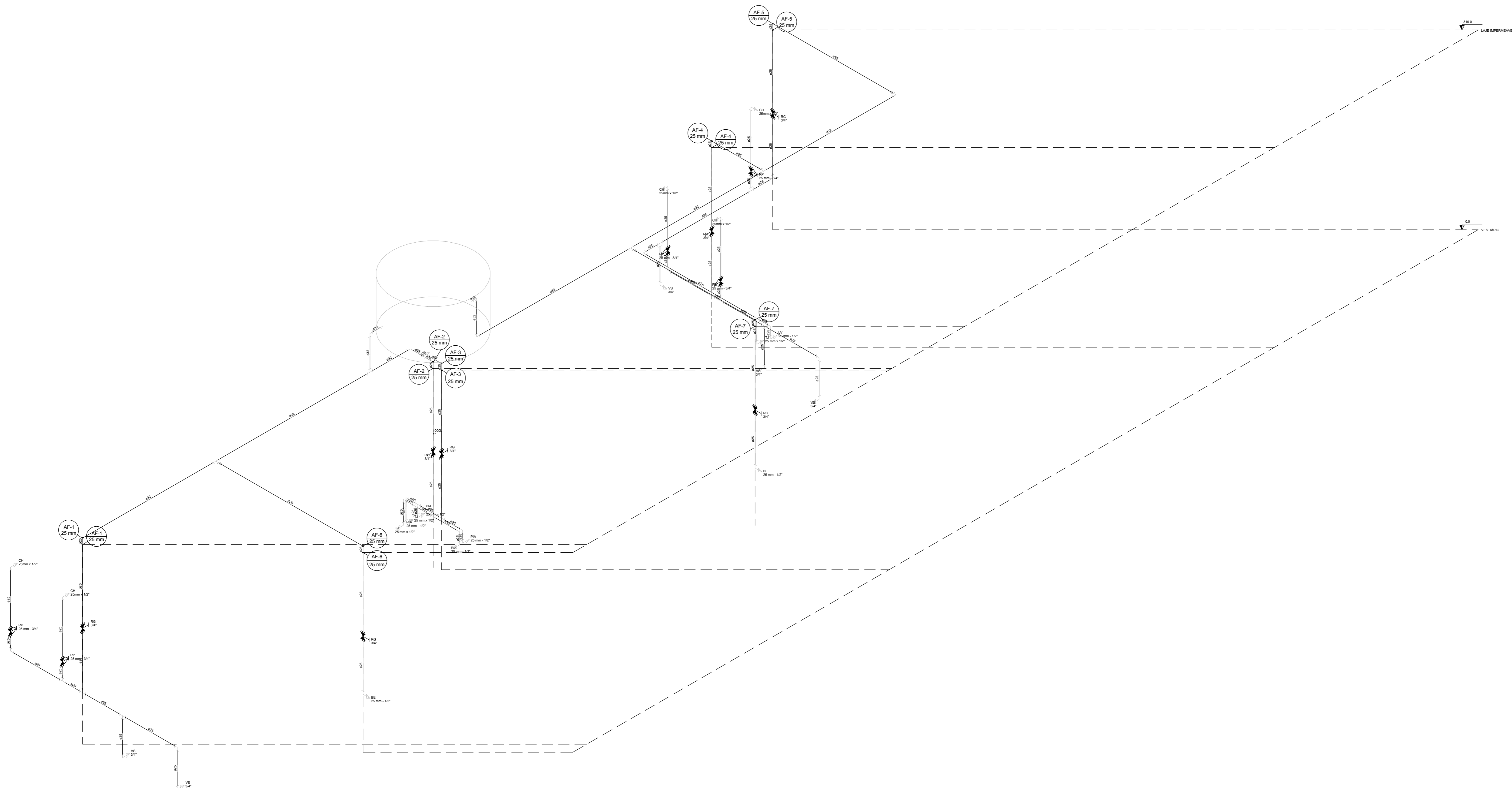
ESQUEMA ISOMÉTRICO HIDRÁULICO ESCALA.....1/25
