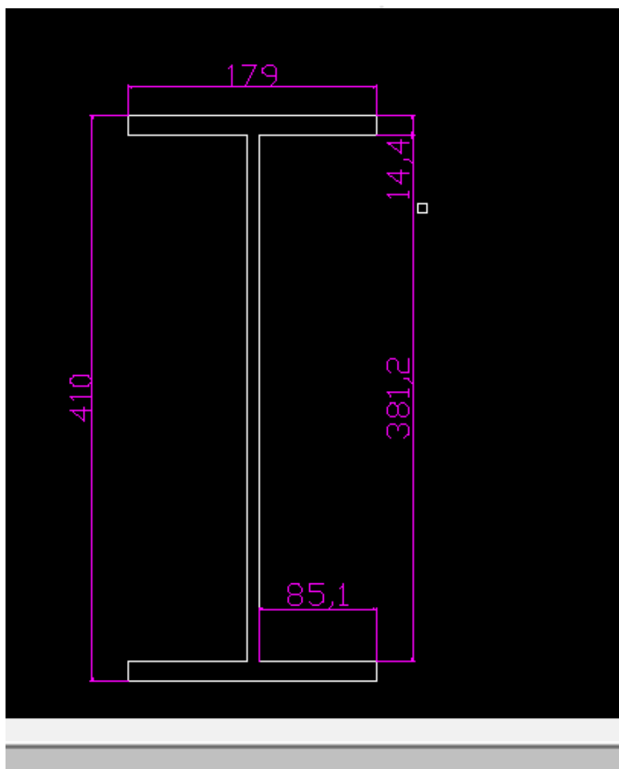
Figura 6- Dimensionamento perfil I
