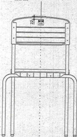
IDENTIFICAÇÃO CENTRALIZADA EM RELAÇÃO AO ENCOSTO
