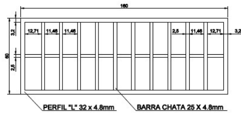
DETALHAMENTO DO GRADIL
