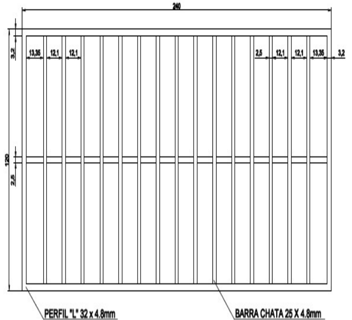
DETALHAMENTO DO GRADIL
